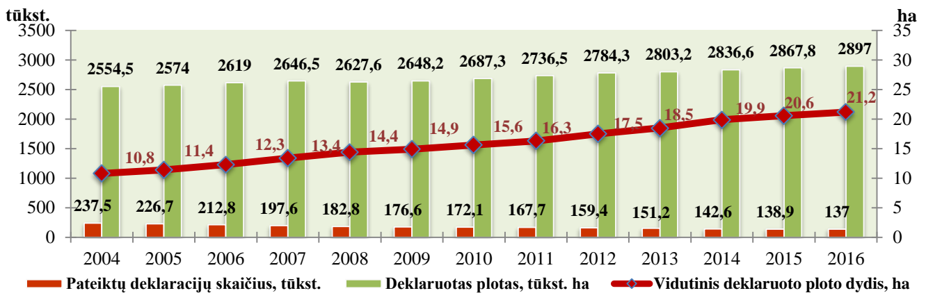
6 pav. Pateiktų deklaracijų skaičius, bendras deklaruotas plotas, vidutinis deklaruoto ploto dydis
